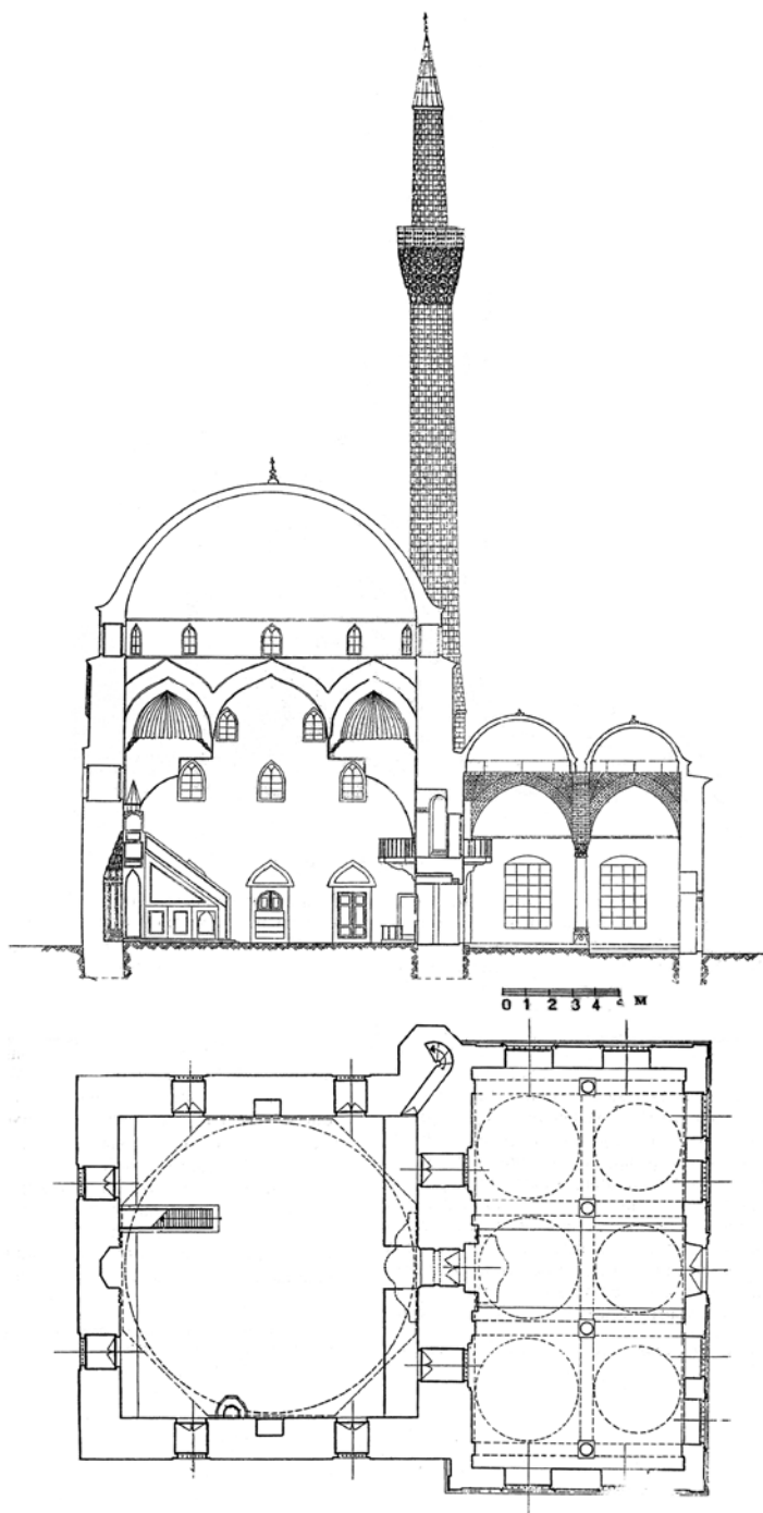
Сл. 3. Основа и пресек на Јени џамија (К. Томовски) fig. 3 - Plan and cross section, according to K. Tomovski
